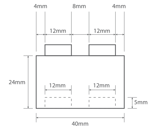
End Elevation
